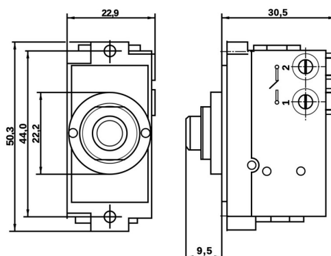
Bouton poussoir, dimensions en mm
